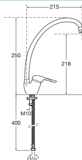
Dibujo técnico
